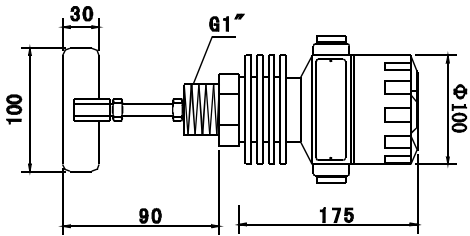
WD-UZK-249G0A/B/C 【丝口连接高温型】
