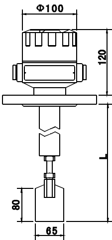
WD-UZK-249C2A/B/C 【轴保护管型】
