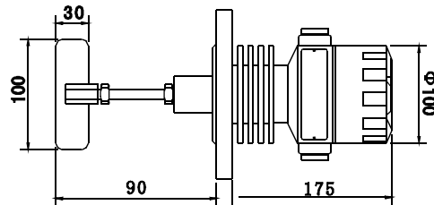
WD-UZK-249G1A/B/C 【法兰连接高温型】
