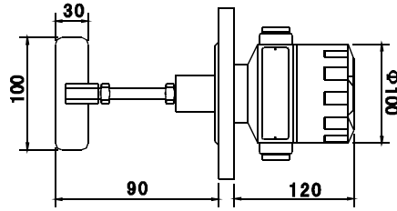
WD-UZK-249C1A/B/C 【法兰型】
