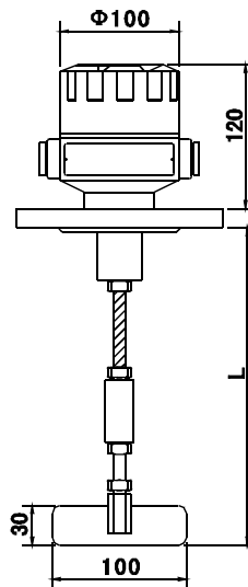
WD-UZK-249C3A/B/C 【轴长可调型】
