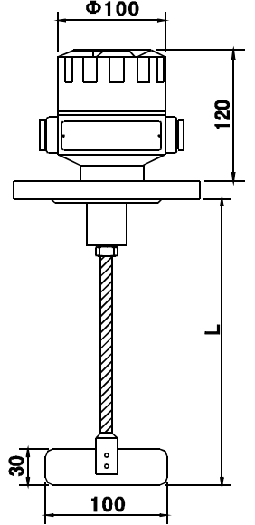
WD-UZK-249C4A/B/C 【钢索型】
