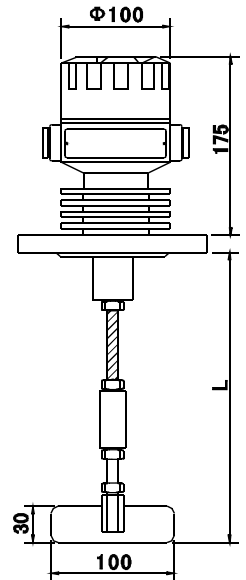
WD-UZK-249G3A/B/C 【高温轴长可调型】
