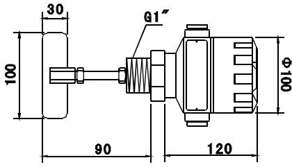
WD-UZK-249C0A/B/C 【丝口型】
