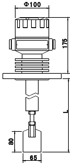
WD-UZK-249G2A/B/C 【高温轴保护管型】
